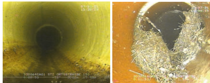
Anschlussleitung Hs.Nr. 6
